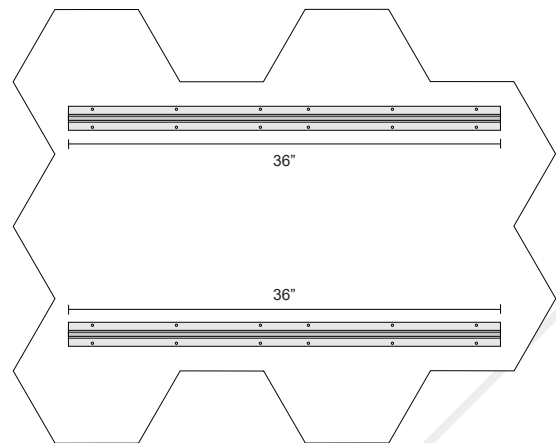
10-Diamond Cluster
